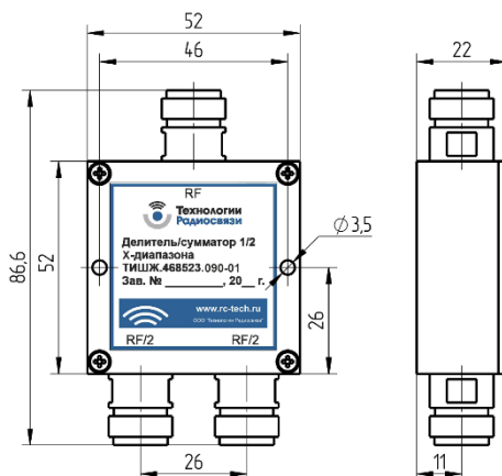
Рисунок – Общий вид изделия.
